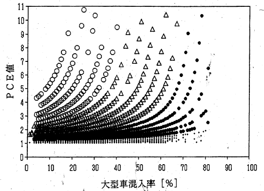
図-7 観測された PCE 値の分布 (東名下り 51.69 kp)
