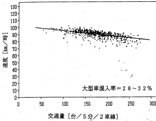
図-2 速度と交通量の関係 (東名下り 51.69 kp)
