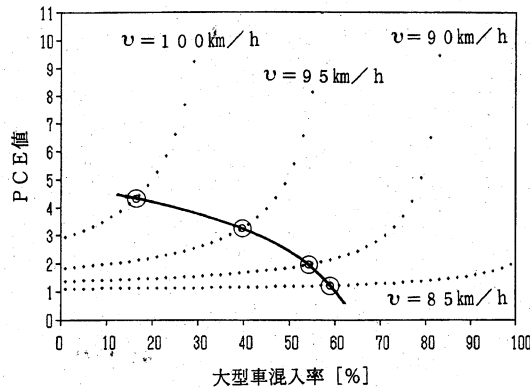
図-6 PCE と大型車混入率の関係 (東名下り 51.69 kp)
