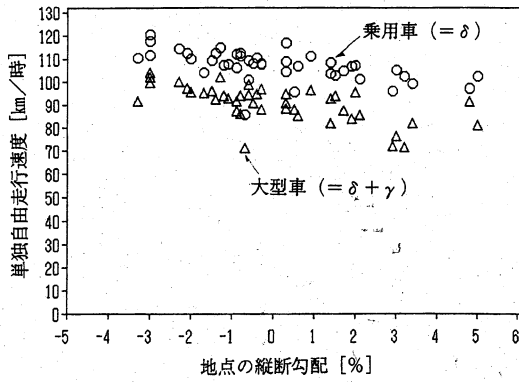
図-5 乗用車および大型車の単独自由走行速度と当該地点の縦断勾配との関係
