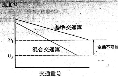
図-8 PCEの定義不可能な領域
