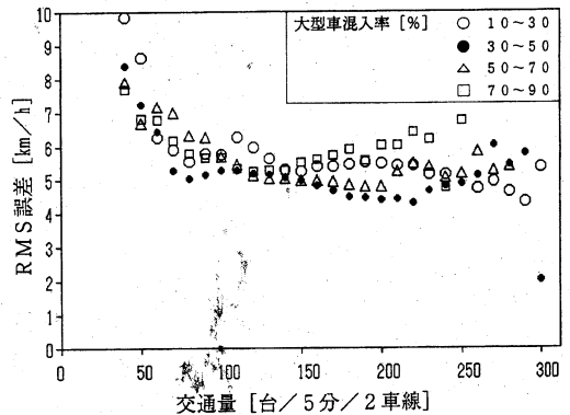
図-12 全地点における交通量と大型車混入率のグループ別のRMS誤差
