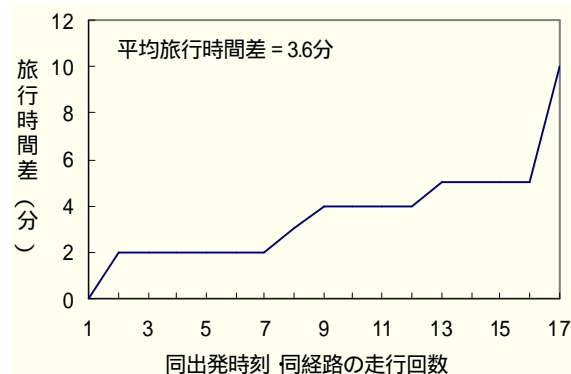
図 4 同出発時刻・同経路における旅行時間差
