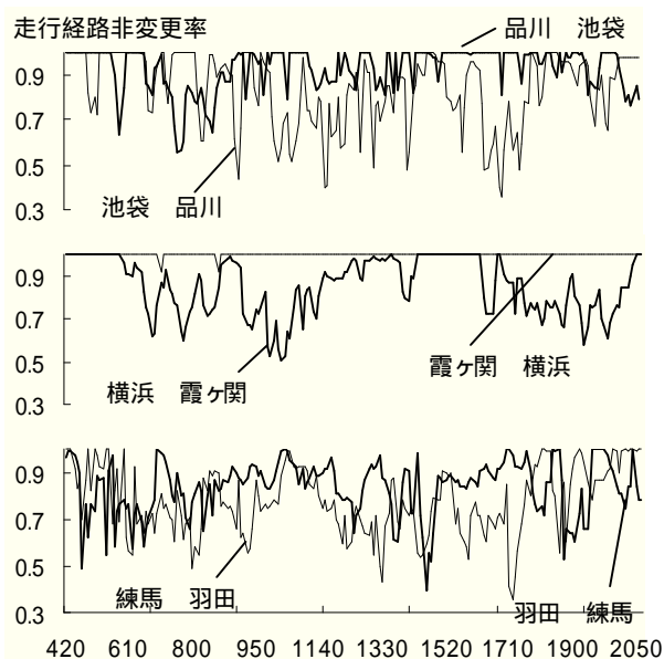
図 7 ODペア別走行経路非変更率
