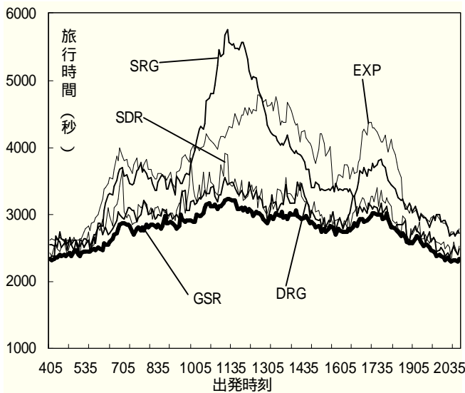
図 5 池袋から品川までの旅行時間図
