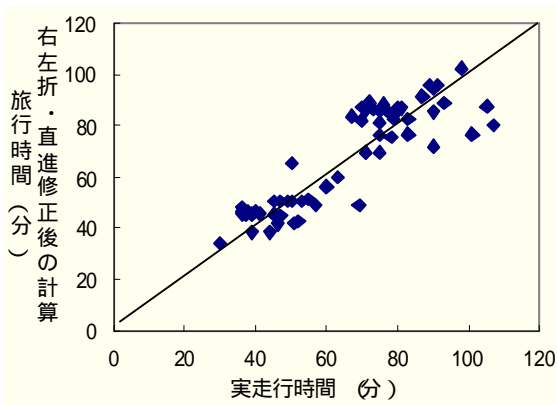
図 3 旅行時間の計算値と実走行値の関係
