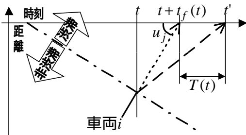
図-6 渋滞・非渋滞の時間と距離との概念図
