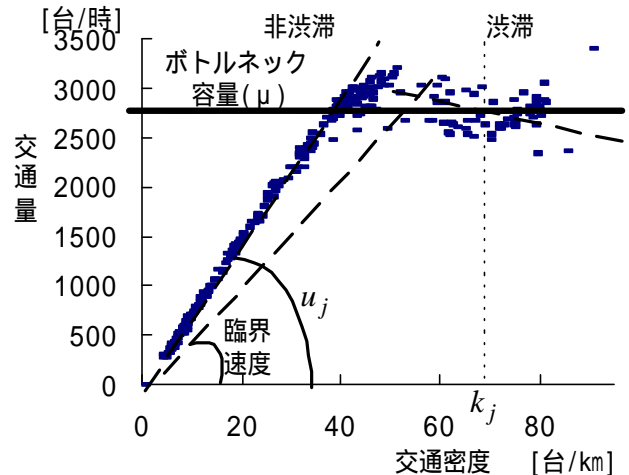
図-5 5.00kp 地点における交通量-密度相関図
