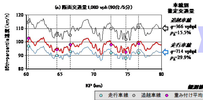
道路線形による通行速度の空間変動の様子がわかる。
