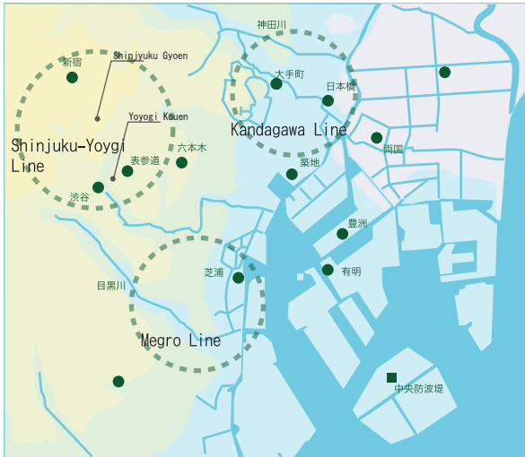
雨水排管を利用したネットワーク
